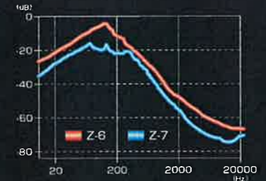
イヤースペースには、風切音の浸入を防ぐ着脱可能なイヤークッションを装着。パッドを取り外したイヤースペースの樹脂プレートにはパンチング加工を施し、内部での音の反響を防ぐ効果をもたらす。
