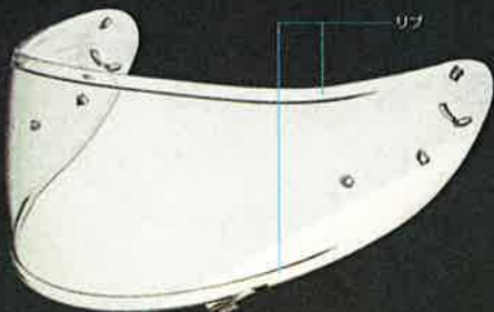
新開発CWR-1シールド。PINLOCK®対応はもちろん、上下にPINLOCK® fog-free sheetの厚みに相当するリブを設け、シールドの装着性を高めると共にシールド全体の剛性も高めている。
